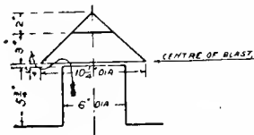
Fig. 4302. THE CONE CAP.
